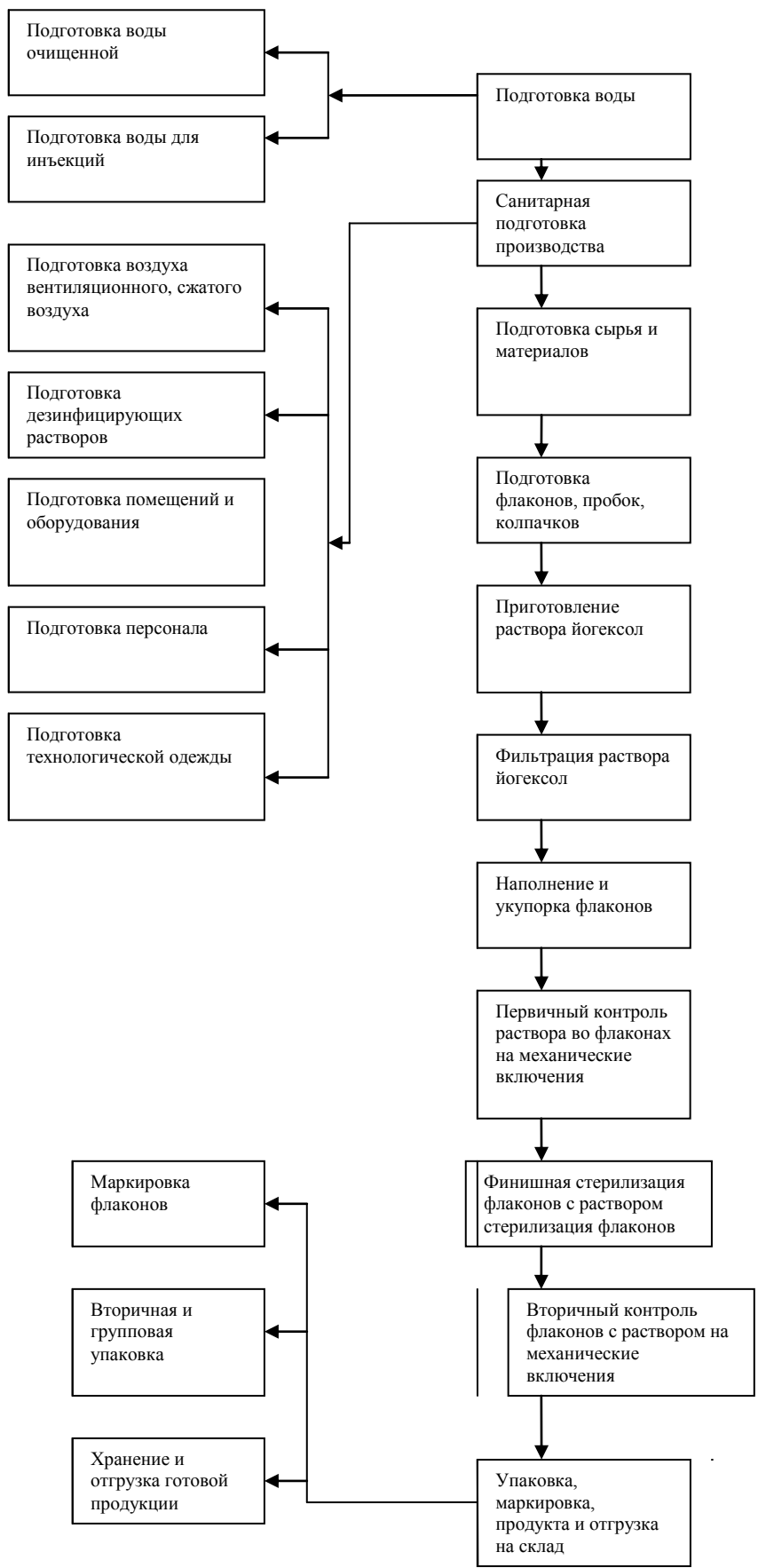
Рис. 1. Технологическая схема производства йогексол
